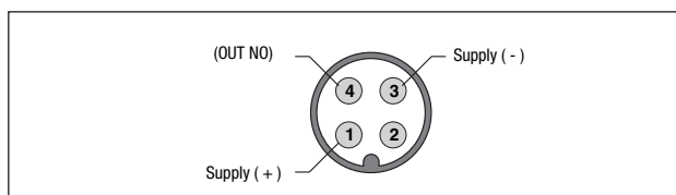
M12 - NO
