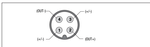
M12 - NO/NC
