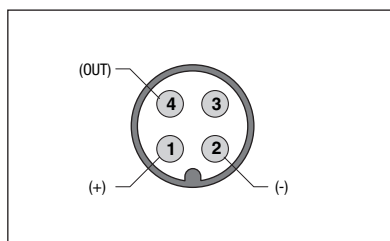
M12 - NO
